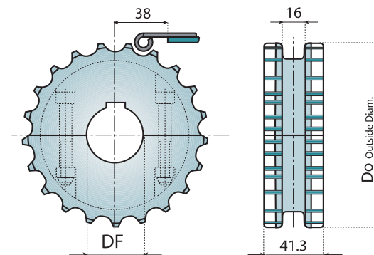
分体式主动轮 (机加工) SPLIT SPROCKET (MACHINED)
