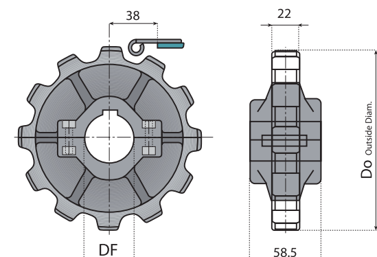
分体式主动轮 (注塑) SPLIT SPROCKET (INJECTION)
