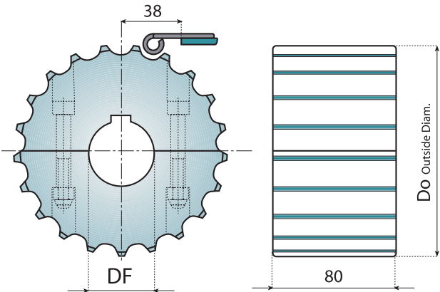
分体式主动轮 (机加工) SPLIT SPROCKET ( MACHINED )
