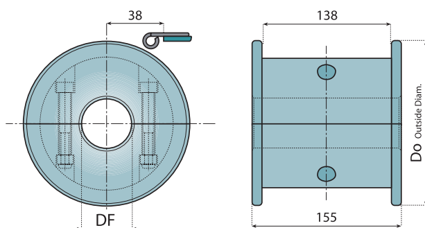
分体式从动轮（机加工） SPLIT IDLER WHEEL ( MACHINED )
