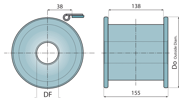
整体式从动轮（机加工） SINGLE PIECE IDLER WHEEL ( MACHINED )
