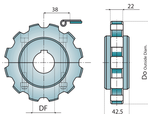
分体式主动轮 (机加工) SPLIT SPROCKET ( MACHINED )
